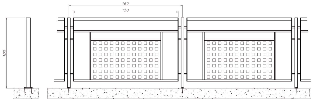
Valla horizontal sobre terreno duro
